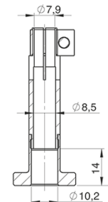
SCHNITT A-A
